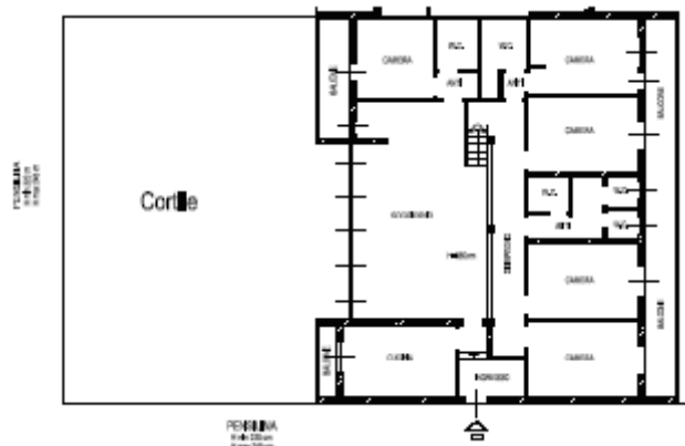
Pianta di Casa Cedro
